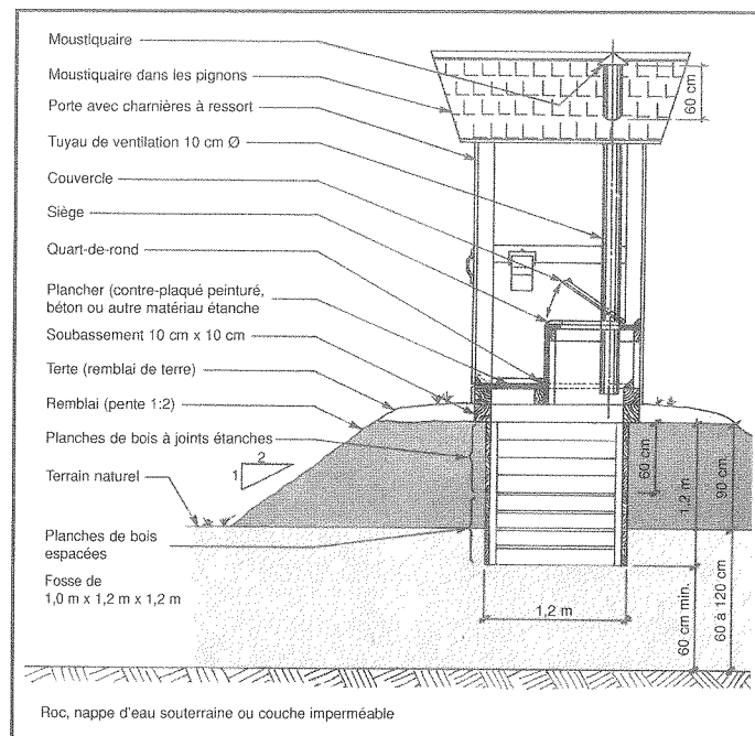
Figure C.62 Détails de construction du cabinet à fosse sèche
