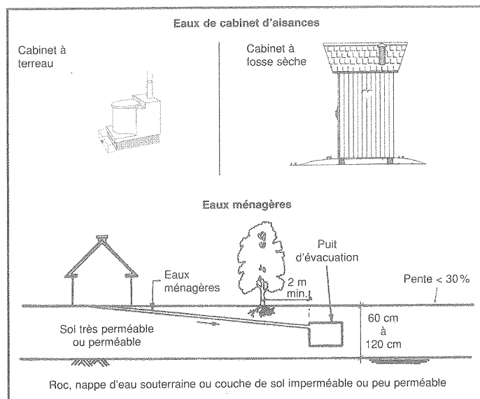
Figure C.61 Le cabinet à fosse sèche ou à terreau et le puits d'évacuation
